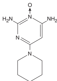
Minoxidil
