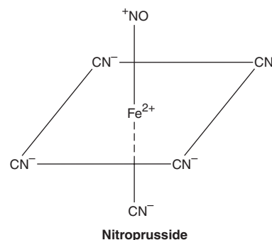
Nitroprusside
