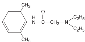
Lidocaine
