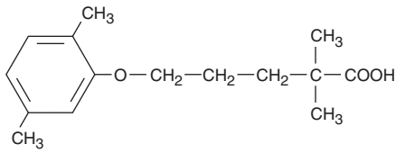
Gemfibrozil
