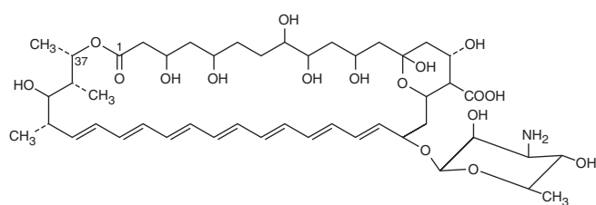
Amphotericin B
