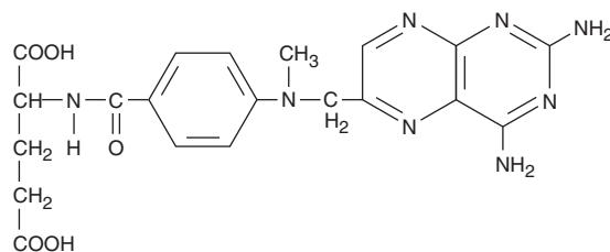
Methotrexate
