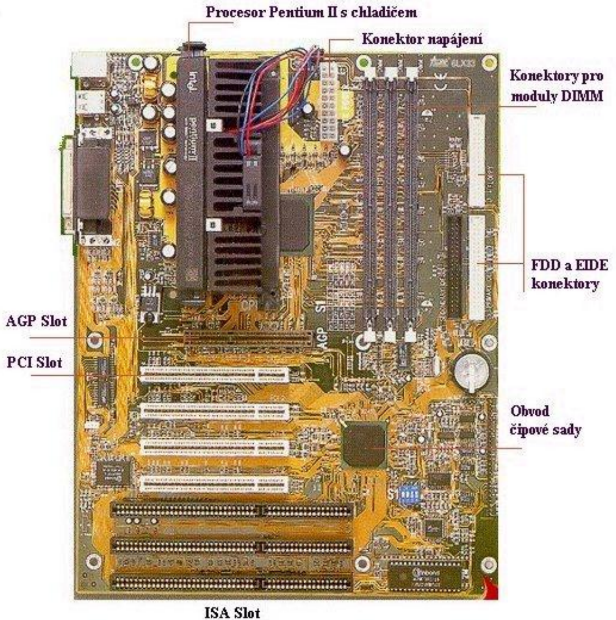
Základní deska pro procesor Intel Pentium II
