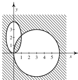
obr. 1.1 Definiční obor funkce f
