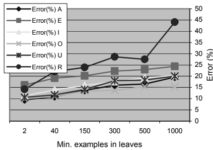
Fig. 2. DT error on different pruning parameters
